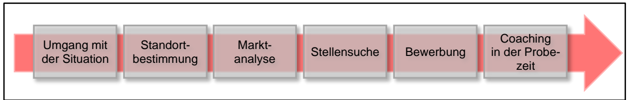
Abbildung 1: Gesamtprozess Outplacement
